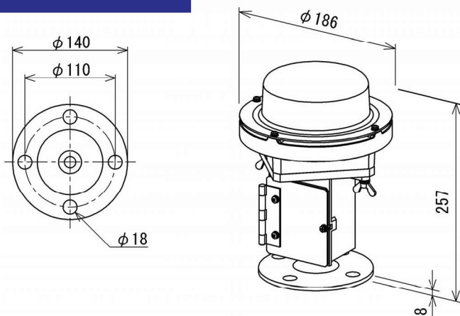
OM-7LC型外形図
