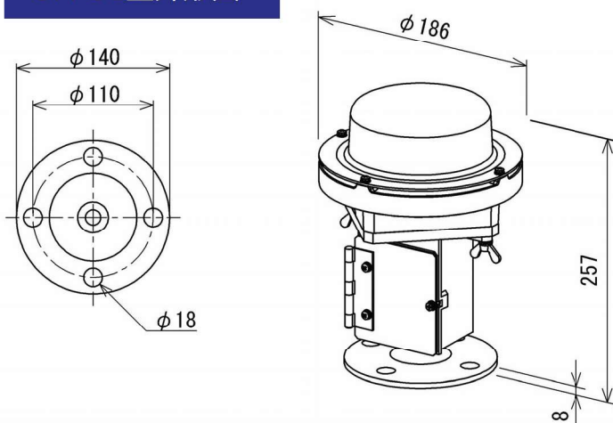
OM-3C型外形図
